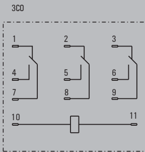
线路布局图 引脚俯视图 尺寸为mm
